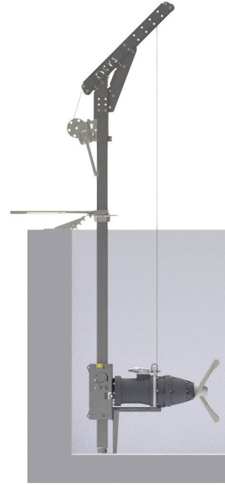
Standart Yerleşim Standart positioning
