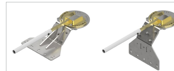
B1 Tip ve B2 Tip Duvar Sabitleyici ve Rotasyon Kolu Type 2A and Type 2B wall mounting
