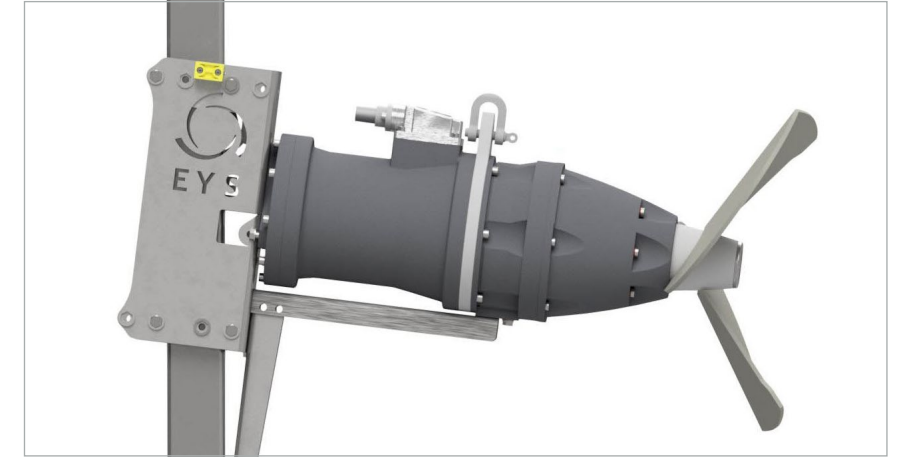
Zemine çöken katmanlar için -7° aşağı eğimli yerleşim Bottom layer solve / -7°
