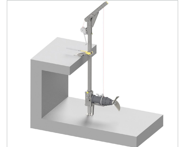
Hareketli platformun biyogaz havuzları içerisindeki yerleşimi Rotatable platform positioning in biogas pits
