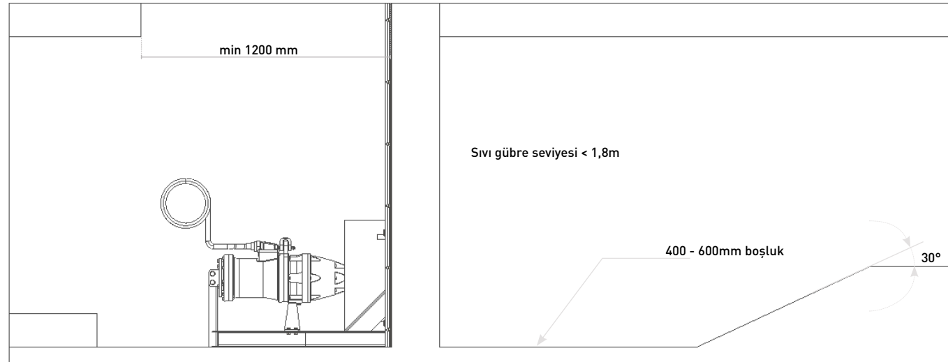
Dalgıç karıştırıcıların slalom tip havuzlar ve kanallar içerisindeki yerleşimi Submersible agitators positioning in slalom type pits and ducts
